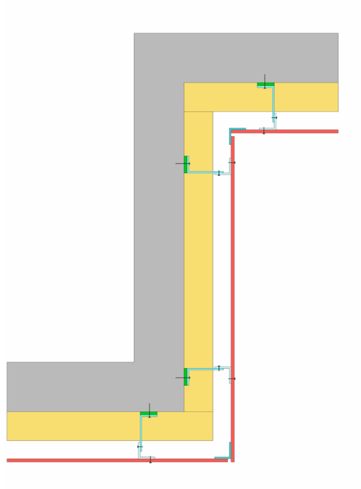
Abbildung 8 - Außen-/Innenecke mit hinterlegtem Profil
