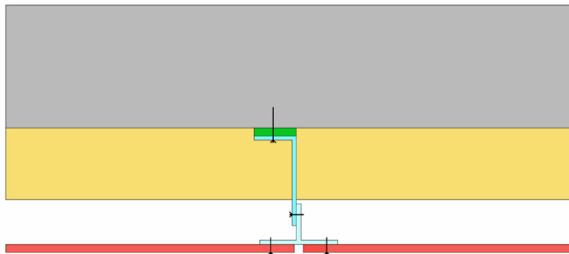
Abbildung 6 - Horizontalschnitt
