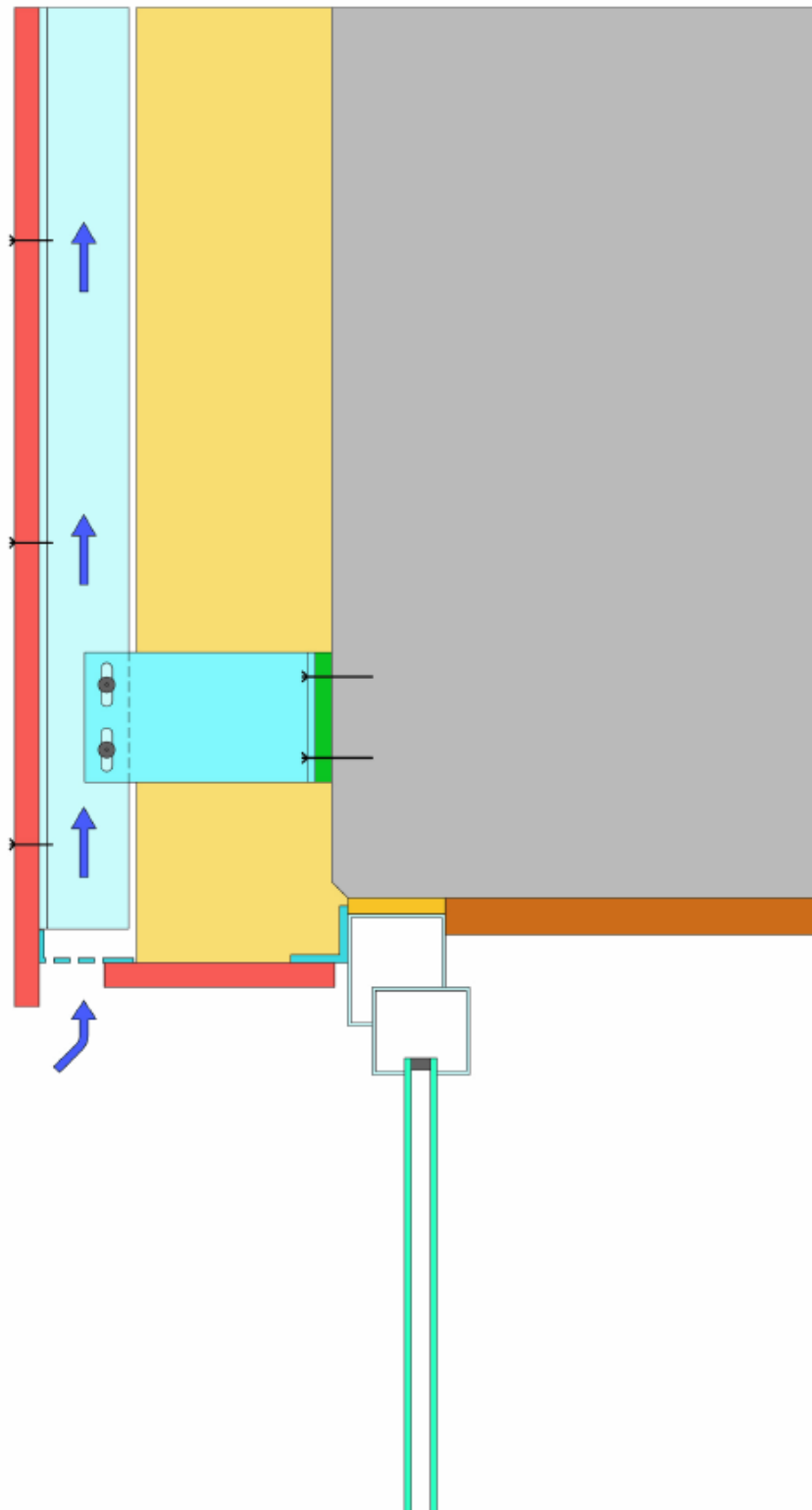
Abbildung 12 - Unter-/Oberseitiger Anschluss (Fenstersturz)
