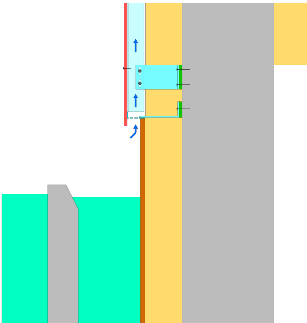
Abbildung 7 - Unterer Fassadenabschluss mit Lüftungsgitter
